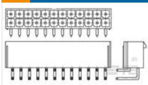
TE 系列/零件编号1586042-8 8P VAL-U-LOK R/A HDR V0
