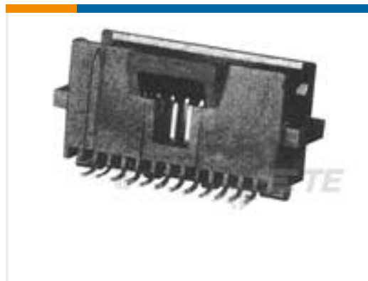
TE 系列/零件编号6-104549- 1 12 SYS50 S/M HDR DRST SHRDSN
