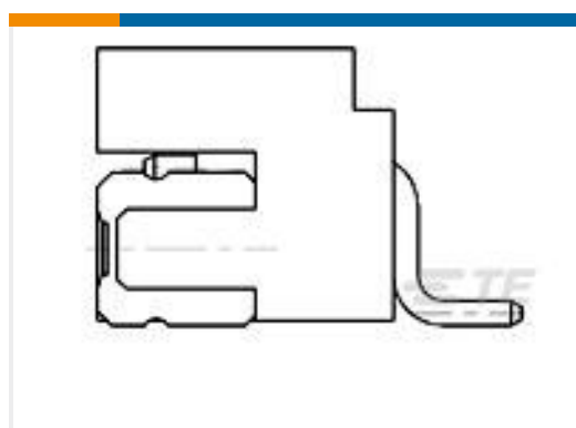
TE 系列/零件编号1- 1734827-4 2.0 WTB HDR .5 SQ RA SMT 14P
