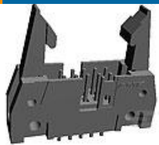
TE 系列/零件编号5746443-8 A/L UNIV HDR 34P ACT PIN LG LAT
