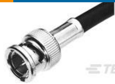
TE 系列/零件编号1- 5413589-6 KIT PLUG 75 OHM BNC HEX CRIMP
