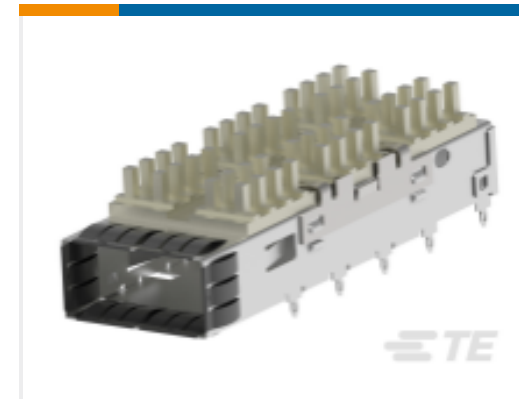
TE 系列/零件编号 1888631-2 Cage Assy SAN Hsink QSFP Thru Bezel
