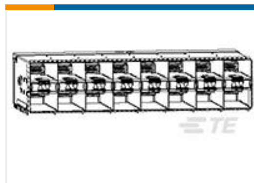
TE 系列/零件编号2198346-7 zSFP+ STACKED 2X8 RECEPTACLE ASSEMBLY
