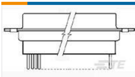
TE 系列/零件编号208869-1 PLUG ASSY,62 POSN, AMPLIMITE
