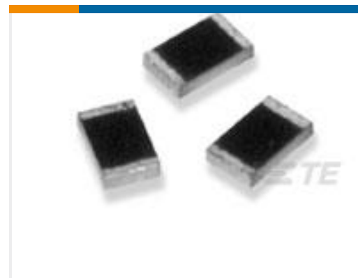
TE 系列/零件编号9- 1879253-5 RP 2B 22R1 0.1% 15PPM 1K RL
