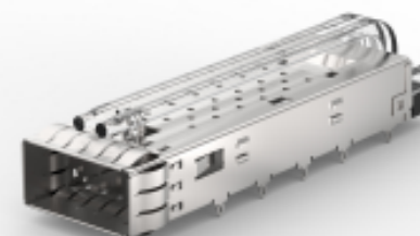
TE 系列/零件编号1888971-4 QSFP TB CAGE ASSY, W /LP, NO HS
