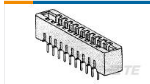
TE 系列/零件编号2-530666-3 CONN LOW PRO 12 POS 156X200C/L
