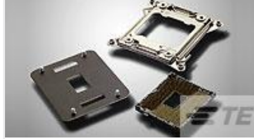
TE 系列/零件编号1554653-1 SOCKET ASSY LGA2011, 0.38Au
