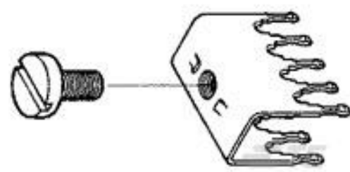
TE 系列/零件编号1-794107-1 22P MINI UMNL R/A HDR ASSY LF
