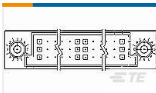
TE 系列/零件编号532433-4 HDI PIN ASSY 3 ROW 105 POS
