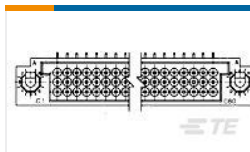
TE 系列/零件编号531133-1 3 ROW BOX PIN 90P R/A UNSEAL
