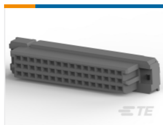
TE 系列/零件编号 5536397-5 ASSY,RECEPT,EURO,TYPE C/2,LEAD
