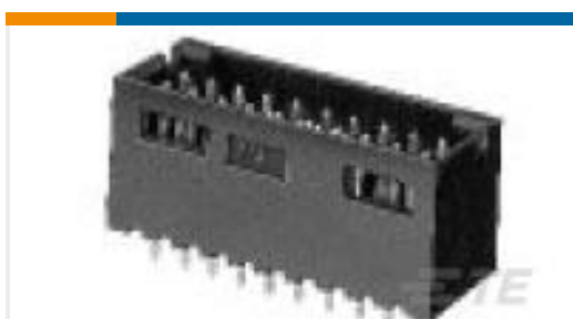
TE 系列/零件编号5223977-1 UNIV. POWER MODULE R /A HEADER
