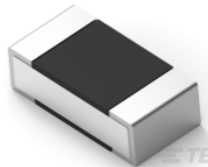
TE 系列/零件编号3- 2176305-3 RP 1E 0.1W 232R 0.1% 25PPM 5K RL
