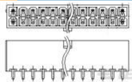
TE 系列/零件编号2- 1658012-4 MSB0.80RC-ASY160FL,-,10, -TY
