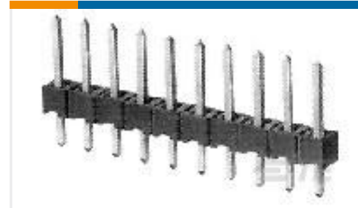
TE 系列/零件编号4-103783-0 80 MODII HDR DRST B/A . 100CL
