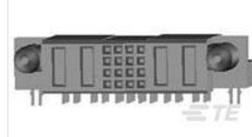
TE 系列/零件编号3- 6450170-1 MBXL R/A RCPT 2P+16S+2P
