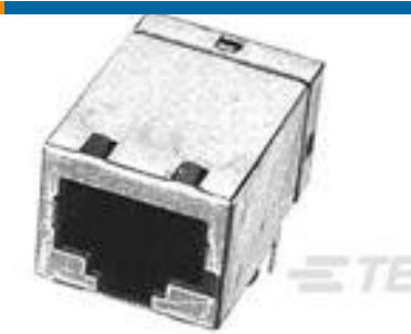
TE 系列/零件编号1- 1734580-4 MOD-Jack,RJ45, 10P10C, SHD LP, 50u" Au
