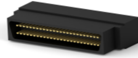
TE 系列/零件编号 5390377-5 50 POS A/P PLUG 25 CL 30AU
