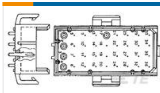
TE 系列/零件编号148059-5 096 EURO TYP C RECP 17MM ASSY
