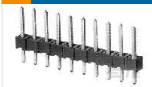
TE 系列/零件编号5536010-5 ASSY,PIN,EUROCARD, TYPE C,LEAD-
