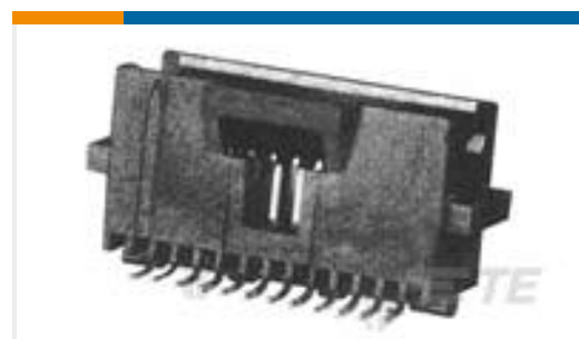
TE 系列/零件编号5120788-1 ZP HS3 DB 06R REC 030P RT PD
