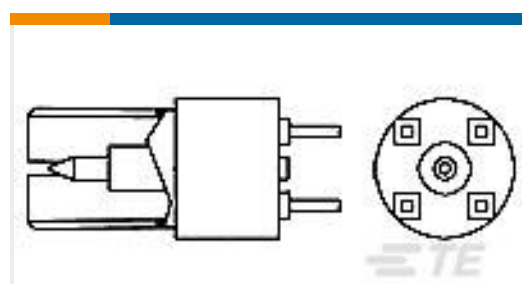
TE 系列/零件编号 1057088-1 3001 7941 00
