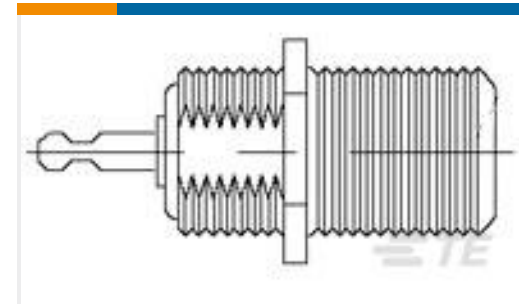
TE 系列/零件编号5-1814823-1 F Type Bulkhead Socket 75 Ohm
