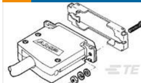
TE 系列/零件编号 1-5499141-0 A/L UNIV HDR 50P RA LG LAT
