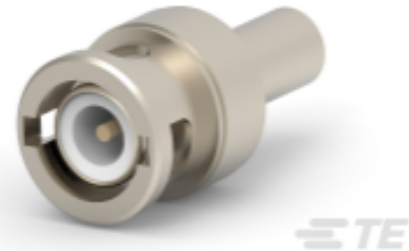
TE 系列/零件编号 5-1634500-1 BNC Str Plg Hex 50Ohm Nickel Plated RG17
