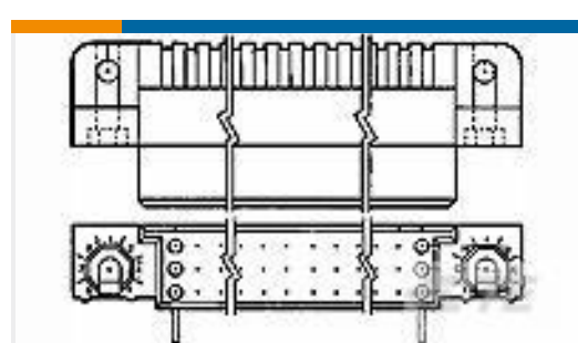
TE 系列/零件编号532834-1 HDI RECP ASSY 3 ROW 165/107
