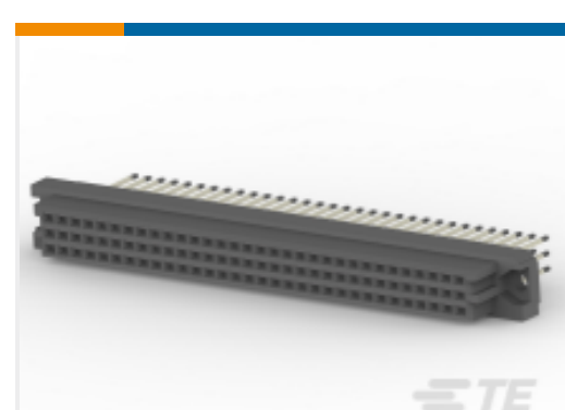
TE 系列/零件编号 5148057-5 ASSY,RECEPTACLE, EUROCARD,TYPE C,LEAD-FRE
