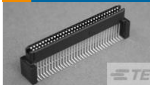
TE 系列/零件编号1-5146896-1 1FHR,64,50A/S,S,C,S14,15
