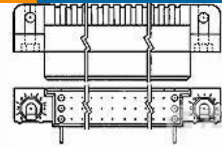
TE 系列/零件编号650809-2 HDI RECP ASSY 3 ROW 180 POS
