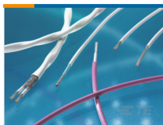
TE 系列/零件编号CW7249- 000 55PC0124-24-0/9-F871
