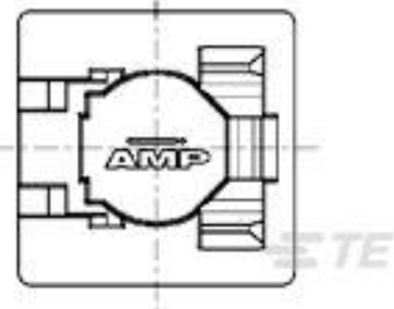
TE 系列/零件编号 188729-1 8P.COVER/SOLD.STOP
