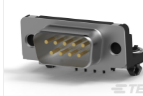
TE 系列/零件编号 5747840-2 HD-20 PLUG RA .318 FMS BD-LK
