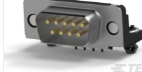
TE 系列/零件编号 5747840-4 HD-20 PLUG RA .318 FMS BD-LK 4
