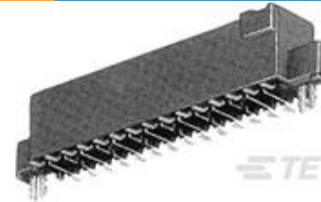
TE 系列/零件编号1-104652-0 100 50/50 GRID DRST SFMNT RCPT
