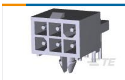
TE 系列/零件编号1-770969- 1 06P MINI UMNL R/A HDR ASSY LF
