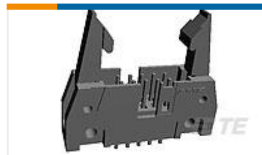
TE 系列/零件编号5102321-1 A/L UNIV HDR 10P VERT LG LAT
