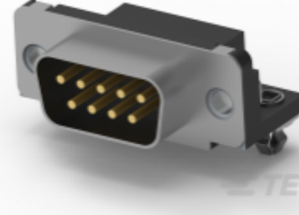
TE 系列/零件编号 5788792-2
