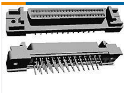
TE 系列/零件编号5749069-9 100 50SR VERT RCPT ASSY
