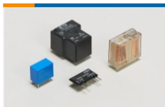
功率继电器(30)
