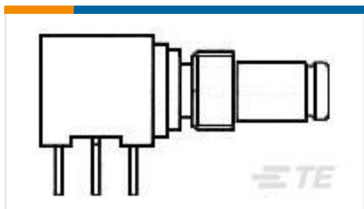
TE 系列/零件编号1460060-1 1.0/2.3 R/A PCB JACK, 50 OHM
