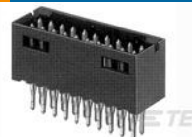
TE 系列/零件编号 102699-3 08 MODII HDR DRST SHRD A/PIN
