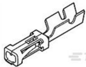
TE 系列/零件编号1-87756-1 MOD IV RECP PLTD 50 SEL
