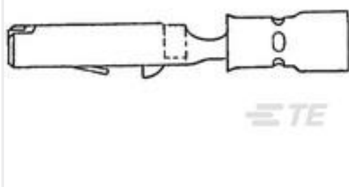
TE 系列/零件编号329317 TERMINAL,LANCELOK N 24-22
