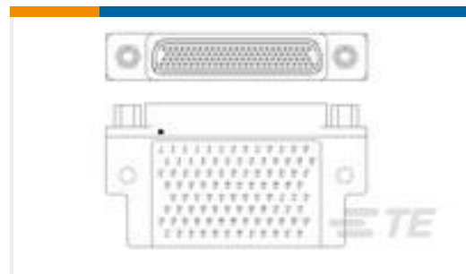
TE 系列/零件编号 1532265-2 M83513/15-H01CP = MCK5-C2-S-100SRT1
