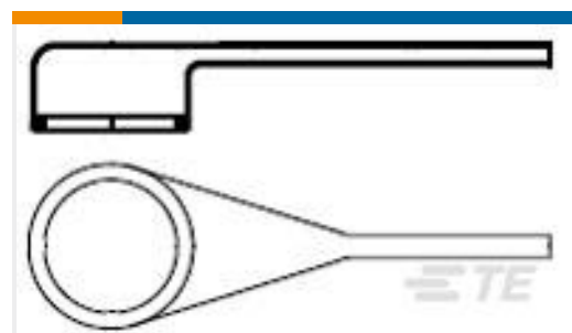
TE 系列/零件编号808472-000 222D932-4-00-0
