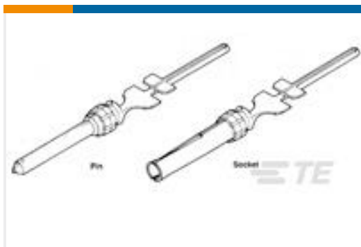
TE 系列/零件编号5-745287-4 20 DF PIN CONTACT DUPLEX/LP
