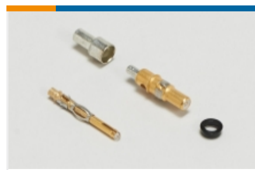
同轴端子(2)
