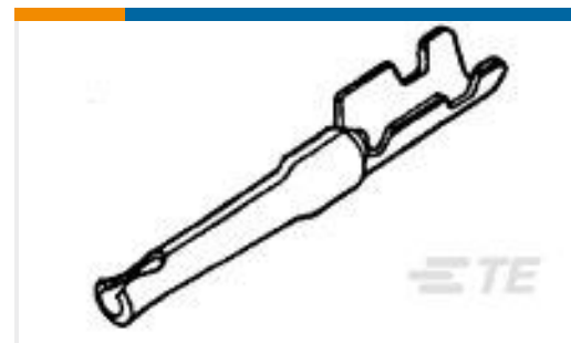
TE 系列/零件编号1658686-1 SOCKET CONTACT,22 DF, STRIP,22-
