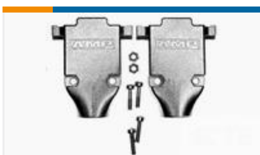
TE 系列/零件编号5748676-5 DIE CAST CBL CLMP KIT, SZ 5
