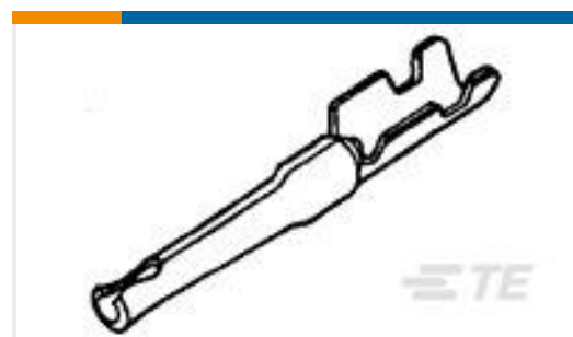
TE 系列/零件编号1658683-1 HDP-22,RCPT,SIZE 3,44 POSN
