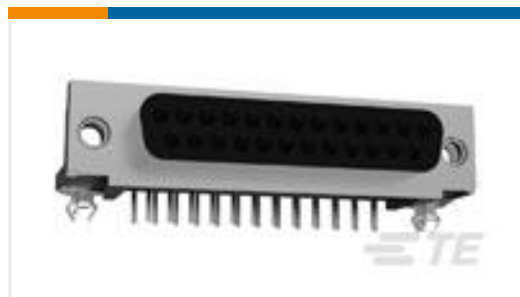
TE 系列/零件编号5747846-4 25 MSFL RCPT RA 318 (IN, FM,BL)
