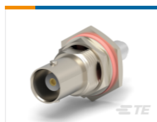
TE 系列/零件编号 5413771-3 JACK BLKHD, COM'L BNC, HEX CRIMP
